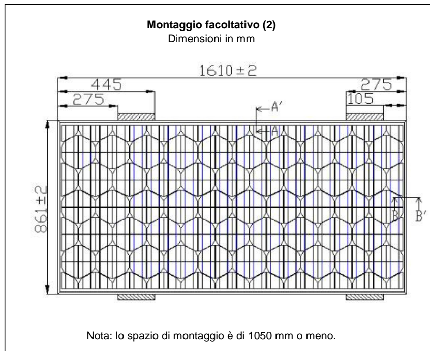
Figura 2-3: Montaggio facoltativo
