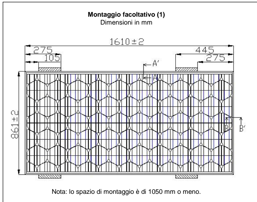
Figura 2-2: Montaggio facoltativo
